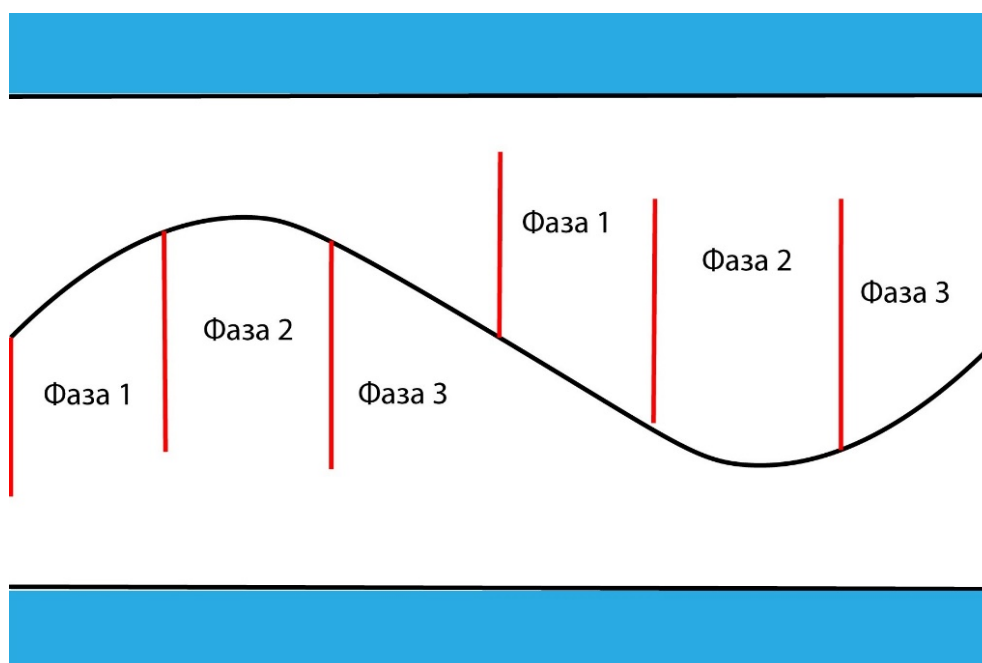
Рис. 2. Траектория передвижения конькобежца на прямой
