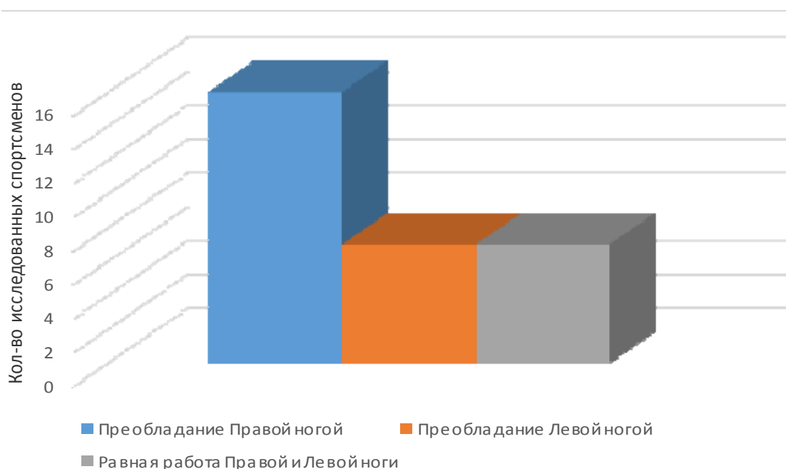
Рис. 4. Распределение спортсменов, специализирующихся на 500, 1 500 и 5 000 м, по доминированию нижних конечностей в фазах свободного проката и одноопорного отталкивания конькобежного шага на прямой
