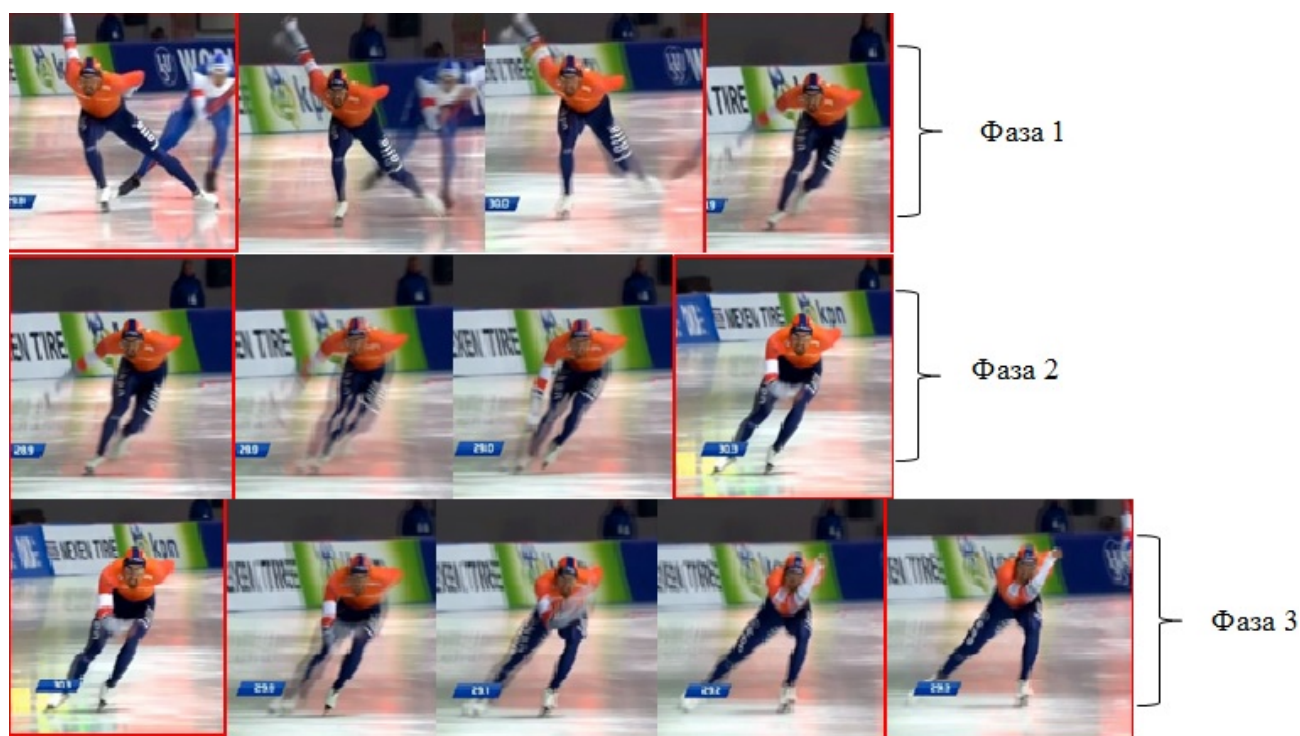
Рис. 1. Фазы движения конькобежца на прямой
