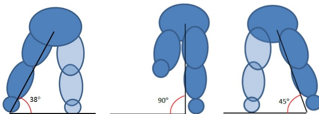
Рис. 3. Смещение ЦМТ конькобежцев с правой и левой опорной ноги при преодолении прямых участков дистанции
