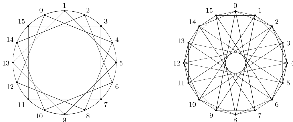
Рис. 1. Циркулянты C(16; 1, 4) и C(16; 1, 2, 7)
