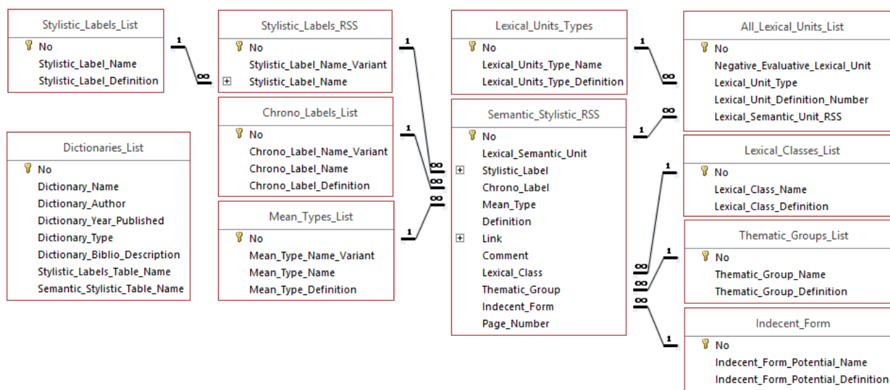
Рис. 1. Схема данных ЛБД ООЛ
