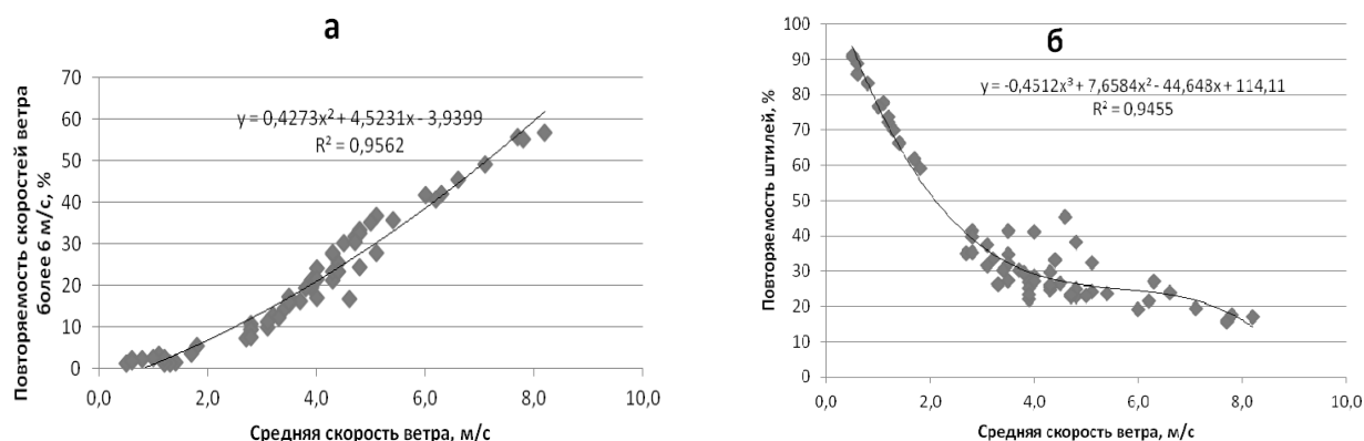
Рис. 7. Зависимость повторяемости скоростей ветра более 6 м/с (а) и штилей (б) от средней месячной скорости ветра, %
