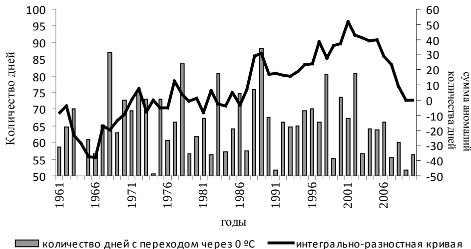
Рис. 3. Динамика числа дней с переходом температуры воздуха через 0^{\circ}\text{C} и интегрально-разностная характеристика ряда для Томской области
