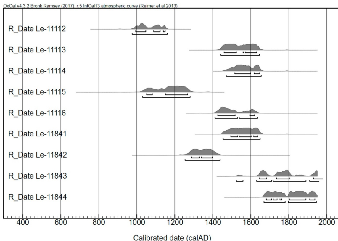
Рис. 2. Радиоуглеродные даты городища «Тоянов городок»
