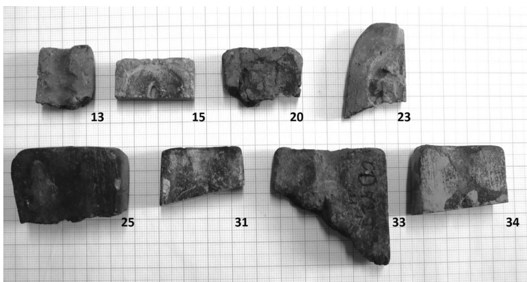
Рис. 3. Объекты, исследованные методом SEM-EDS: фрагменты керамических форм с признаками насыщения углеродом рабочей стороны. На фото указаны порядковые номера объектов
