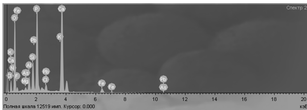
Рис. 8. EDS-спектр: объект № 31, участок 1, спектр 2. Точка снятия спектра соответствует минеральному включению угловатой формы (рис. 7)
