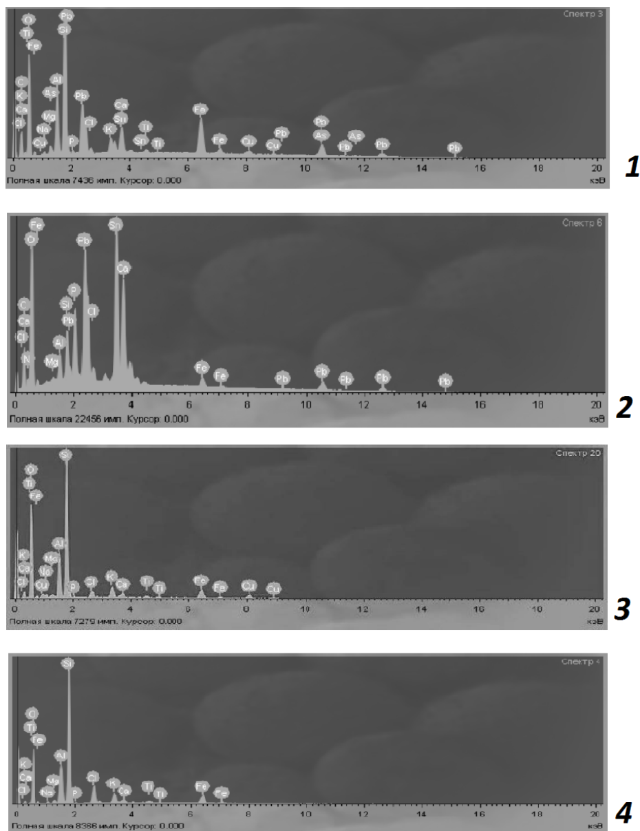
Рис. 6. Спектрограммы: 1 – объект № 13, участок 1, спектр 3. В составе спектра – свинец (Pb), олово (Sn), медь (Cu), мышьяк (As); 2 – объект № 34, участок 1, спектр 6. В составе спектра – свинец (Pb), олово (Sn); 3 – объект № 23, участок 1, спектр 20. В составе спектра – медь (Cu); 4 – объект № 16, участок 1, спектр 4. Элементный состав спектра соответствует стандартному составу глины и керамики
