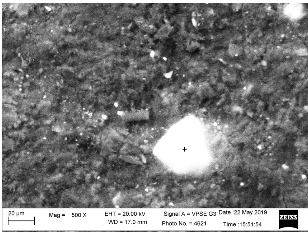
Рис. 7. Электронный скан: объект № 31, участок 1. В центре – включение угловатой формы (+), в составе которого диагностированы высокие концентрации фосфора (P) и кальция (Ca)
