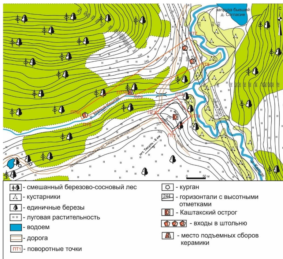
Рис. 2. Ситуационный план окрестностей острога и входов в копи (штолен)
