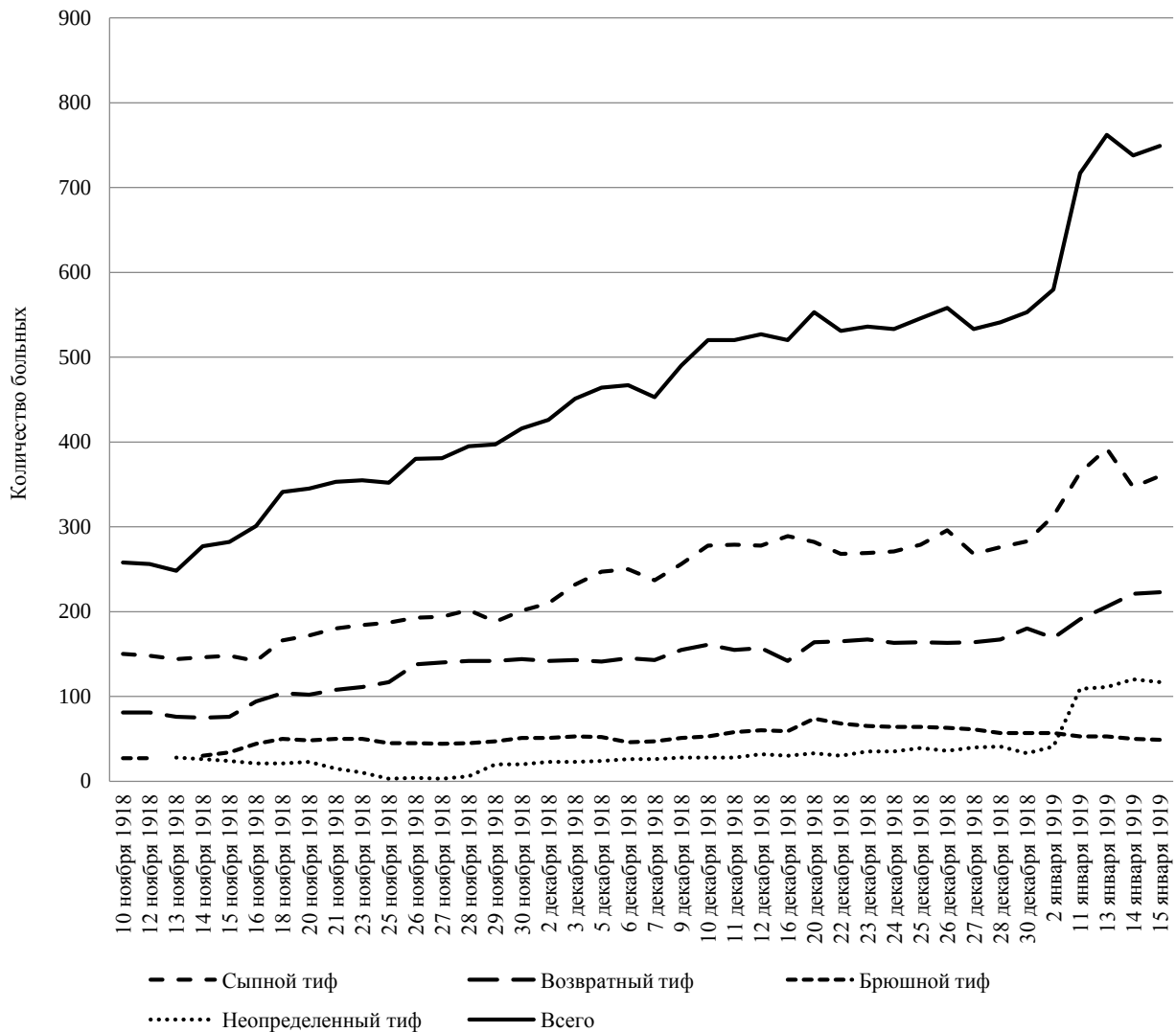
Рис. 2. Структура эпидемии по видам тифа в ноябре 1918 – январе 1919 г. (чел.).
