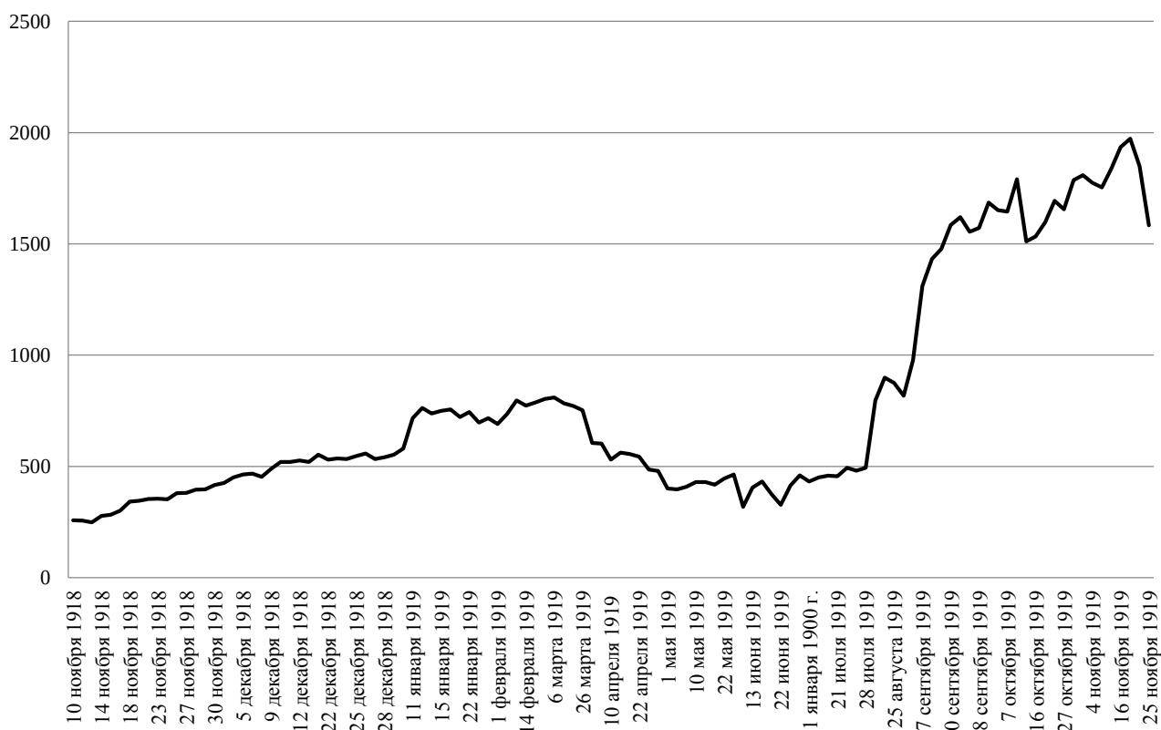
Рис. 1. Количество больных всеми видами тифа в Новониколаевске в ноябре 1918 – ноябре 1919 г. (чел.).
