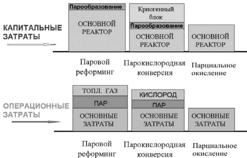
Рис. 4. Сравнение эффективности различных процессов получения синтез-газа
