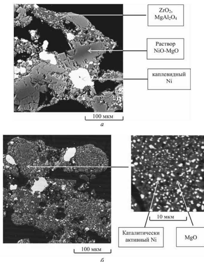
Рис. 3. Микроструктура Ni-Al 2 O 3 -MgO-ZrO 2 -CaO блочного катализатора до (а) и после активации (б)
