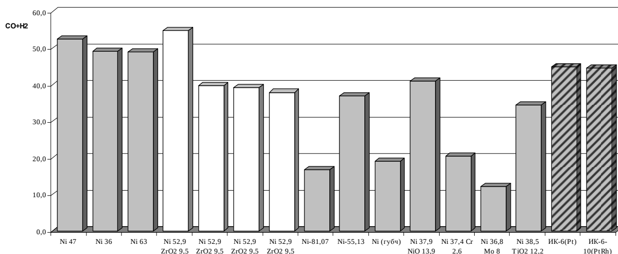
Рис. 2. Концентрация синтез-газа с использованием катализаторов (обозначения соответствуют таблице: заштрихованная область – образцы, разработанные в Институте катализа СО РАН, г. Новосибирск)
