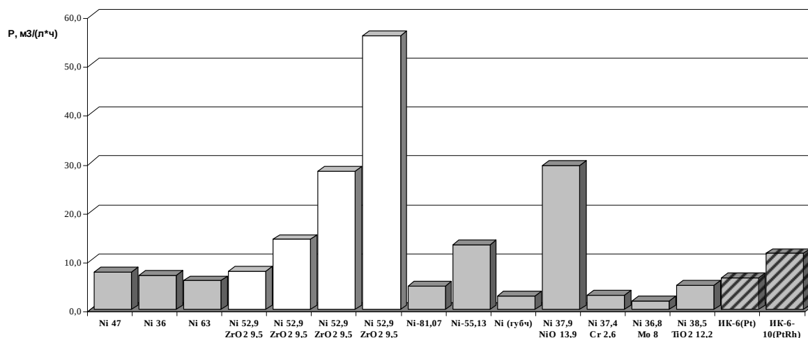
Рис. 1. Производительность по синтез-газу с использованием катализаторов (обозначения соответствуют таблице: заштрихованная область – образцы, разработанные в Институте катализа СО РАН, г. Новосибирск)
