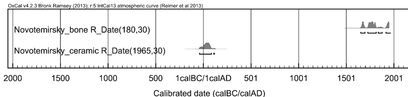
Рис. 7. Вероятностные интервалы калиброванных радиоуглеродных датировок материалов из культурного слоя рудника Новотемирский
