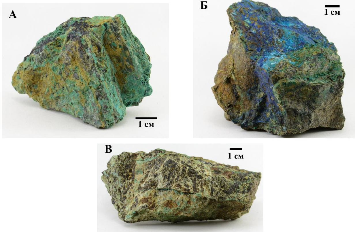
Рис. 5. Типы окисленных медных руд Новотемирского рудника: А – окисленная руда в серпентините (малахит, хризоколл); Б – окисленная руда в серпентините (азурит, малахит, хризоколл), В – медно-магнетитовая руда
