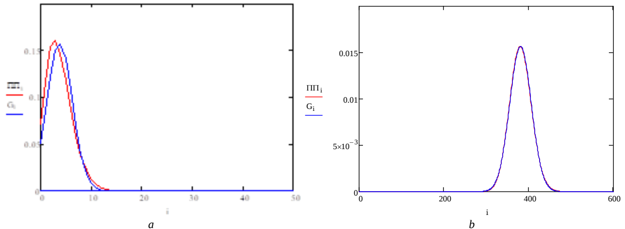
Рис. 4. Изменение числа заявок на орбите для RQ-системы с коллизиями, H -настойчивостью и отказами при H = 0,6 :
