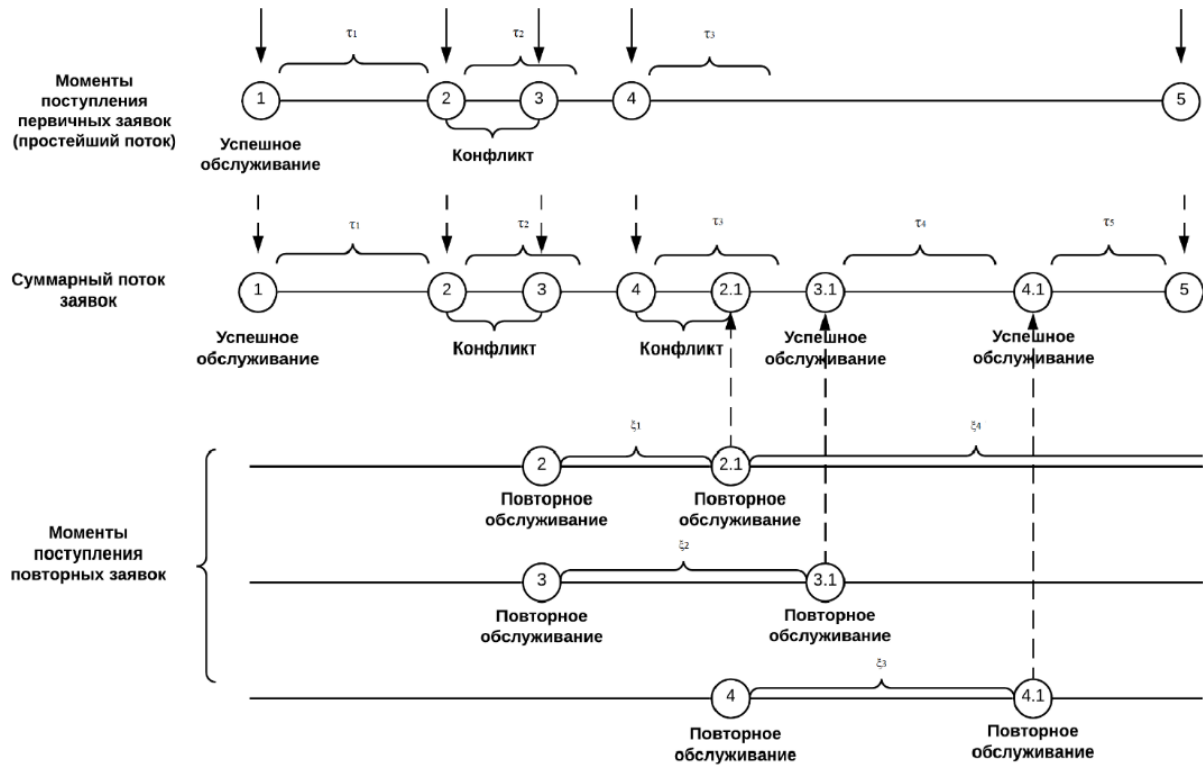
Рис. 1. Схема моделирования суммарного входящего потока заявок
