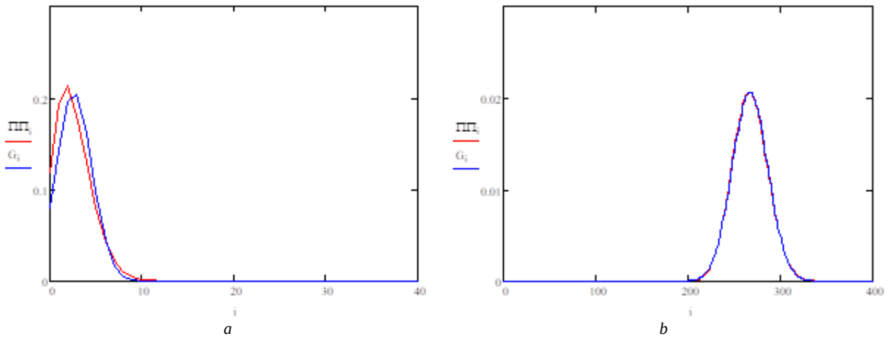
Рис. 3. Изменение числа заявок на орбите для RQ-системы с коллизиями, H -настойчивостью и отказами при H = 0,4 :
