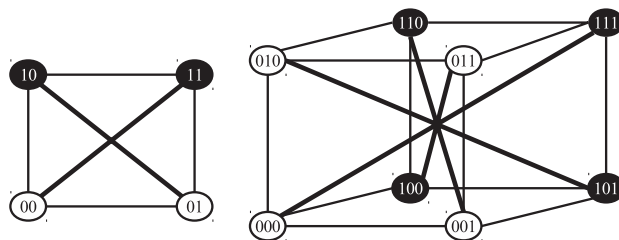
Рис. 2. Минимальные рёберные 1-расширения для Q_2 и Q_3
