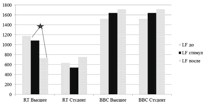
Рис. 7. Различие показателей LF студентов и людей с высшим образованием до, во время и после просмотра ролика RT и ВВС. Здесь и на рис. 8 звездочкой отмечены достоверные различия по критерию Вилкоксона ( p < 0,05 )
