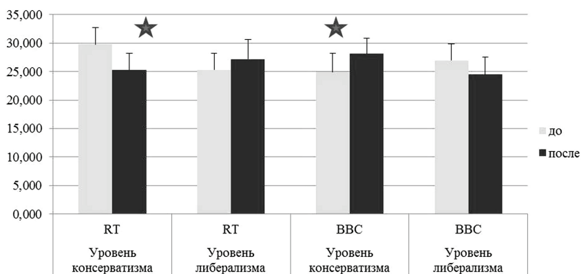
Рис. 3. Различия уровней консерватизма и либерализма до и после информационного воздействия с учетом фактора КОНТЕКСТ (RT – просмотр новостного ролика телеканала RT; ВВС – просмотр новостного ролика телеканала ВВС). Звездочкой отмечены достоверные различия по критерию Вилкоксона ( p < 0,05 )
