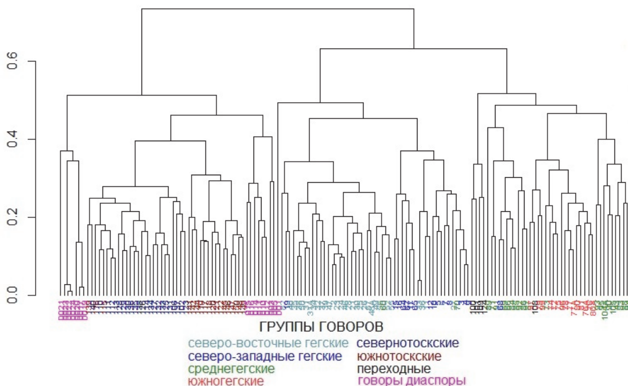
Рис. 5. Кластеризация албанских говоров основного ареала и диаспоры: все признаки
