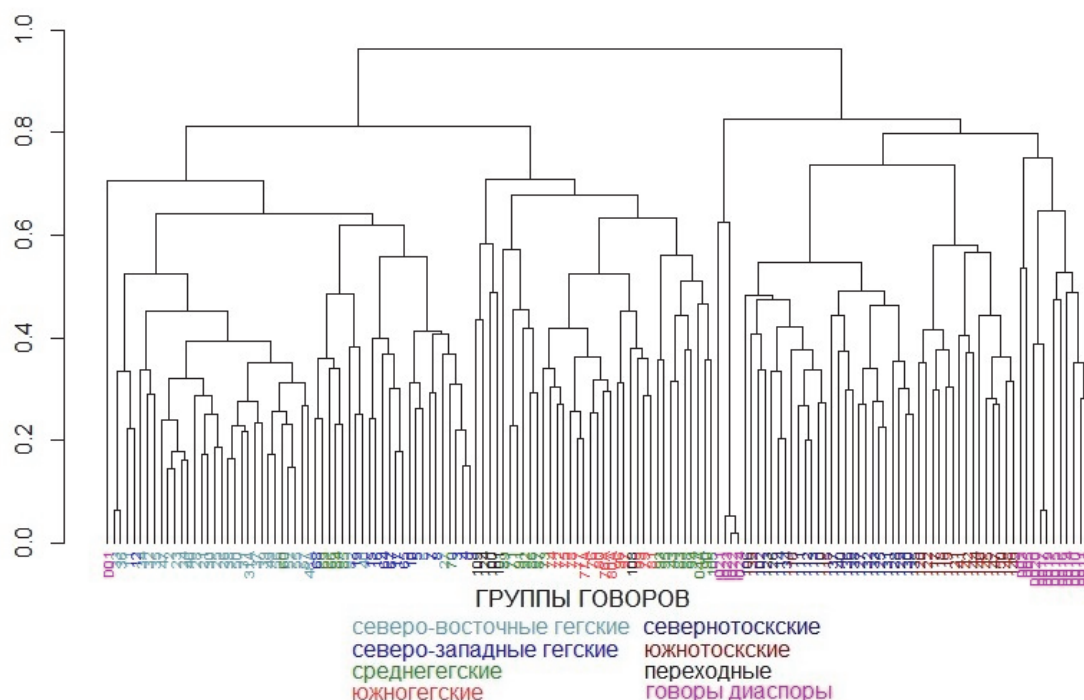
Рис. 6. Кластеризация албанских говоров основного ареала и диаспоры: инновации
