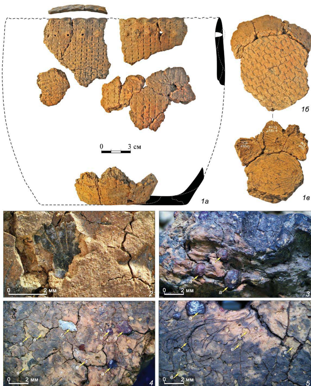
Рис. 5. Керамика поселения Писаная-4. Группа 6. Сосуд б/1. 1а – частичная реконструкция сосуда; 1б – вид внешней поверхности дна; 1в – вид внутренней поверхности дна; 2 – включение раковины в составе ИПС; 3–5 – микрофотографии изломов и поверхностей сосуда, характеризующие состав исходного пластичного сырья и формовочных масс (а – окатанные железистые включения в составе ИПС; б – включения дробленой каменной породы; в – частицы шамота; г – отпечатки шерсти)
