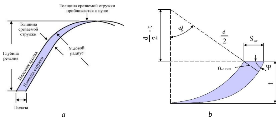
Рис. 3. Схемы определения толщины срезаемой стружки при фрезеровании сферической торцевой фрезой: а – общий вид сечения стружки; б – геометрическая схема
