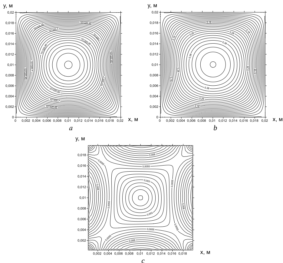
Рис. 3. Стационарное поле давления (a), относительной концентрации паров примесей (b), скорости течения газа (c) в пористом пространстве между металлической пластиной и поверхностью металлокерамической платы ( \Delta = 60 \cdot 10^{-6} м)
