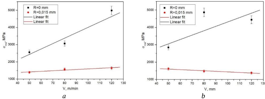
Рис. 9. Зависимость максимальных значений эквивалентных напряжений от скорости резания при фрезеровании заготовки: a – из нержавеющей стали AISI 304 SS; b – из титанового сплава Grade 5 Fig. 9. Maximum equivalent stress as a function of the cutting speed during milling of the workpiece made of: ( a ) AISI 304 SS stainless steel and ( b ) Grade 5 titanium alloy
