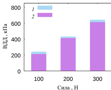
Рис. 4. Гистограмма внутридискового давления при одноосном сжатии с разными силами (1 – экспериментальные данные [26], 2 – данные расчетов по разработанной модели) Fig. 4. Histogram of intradiscal pressure under uniaxial compression with different loads (1, experimental data [26]; and 2, calculated results)
