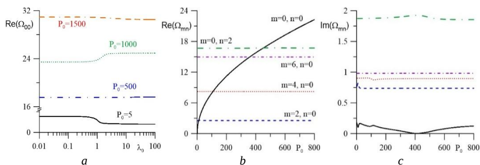
Рис. 3. Зависимость \text{Re}(\Omega) (a, b) и \text{Im}(\Omega) (c) первых гармоник от \lambda_0 и P_0 при b = 1 , R_0 = 5 , k = 1 , \lambda_0 = 10 (b, c), m – азимутальное число, n – волновое число
