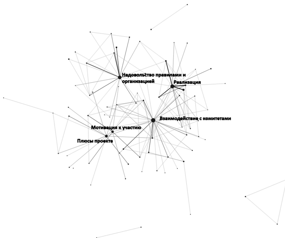
Рис. 1. Граф
