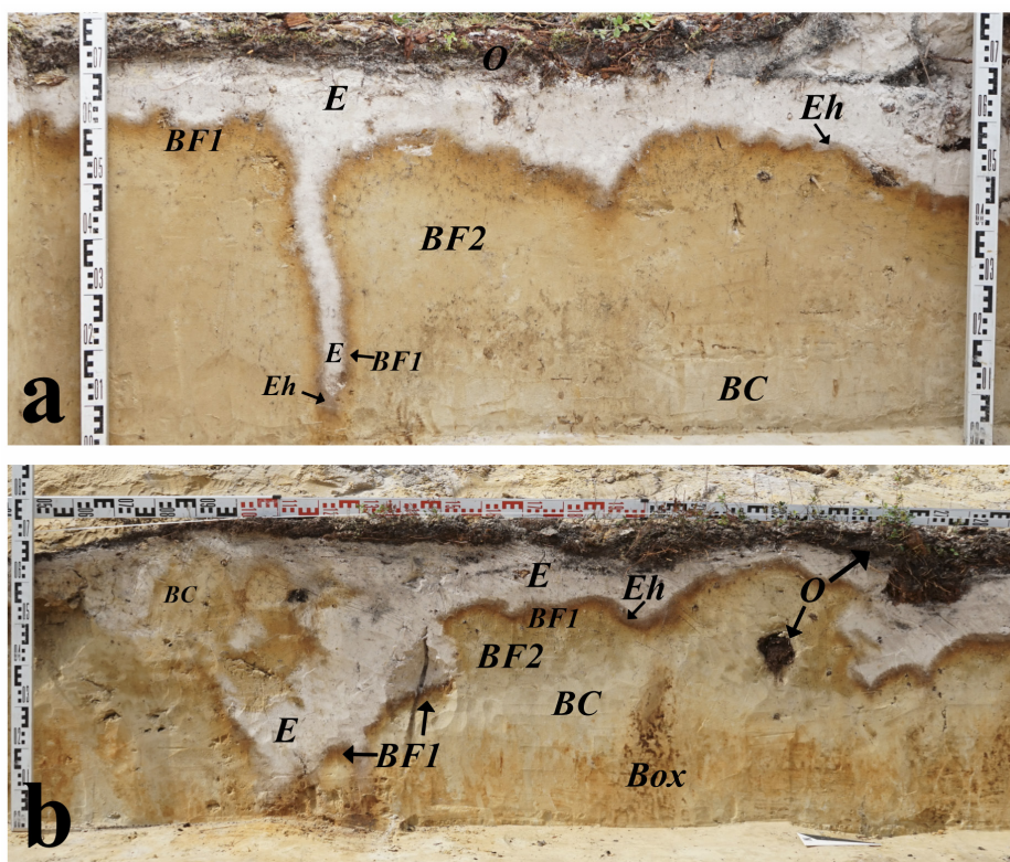
Рис. 2. Горизонты и морфоны профилей изученных почв: a – подзол иллювиально-железистый языковатый на гряде; b – подзол иллювиально-железистый языковатый глееватый в западине [Fig. 2. Horizons and morphons of the studied soil profiles: a - Glossic Albic Podzol (Lamellic) on the ridge; b - Glossic Stagnic Albic Podzol in the depression]
