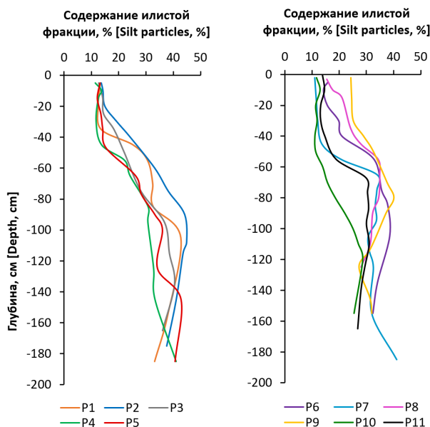
Рис. 2. Распределение илстых частиц (<0,001) по профилю почвенных разрезов 1–11 [Fig. 2. Distribution of silt particles (<0.001) along the soil profiles 1–11]
