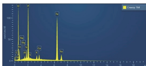
Рис. 1. Отображение химического состава образца на экране РФА-детектора
