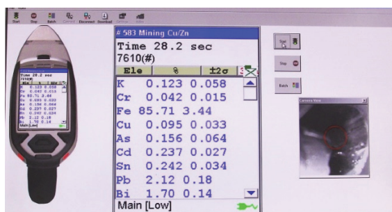
Рис. 1. Отображение химического состава образца на экране РФА-детектора
