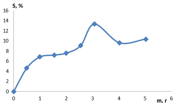
Рис. 1. Влияние массы сорбента на степень поглощения ионов меди
