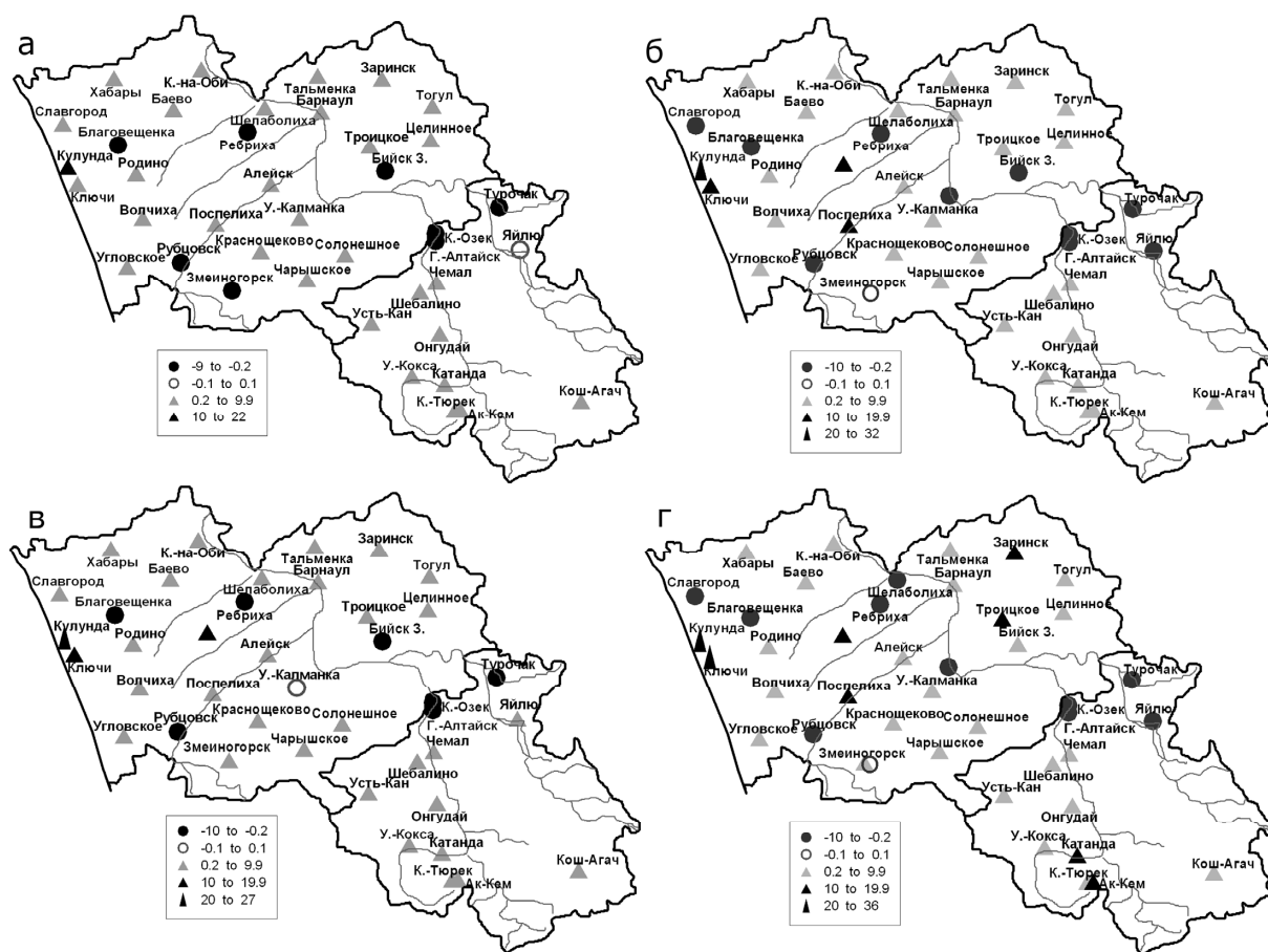
Рис. 3. Пространственное распределение в Алтайском регионе аномалий годовых сумм осадков (%), для периодов: а – 1976–2013 гг.; б – 1991–2013 гг.; в – 1981–2010 гг.; з – 1998–2013 гг.
