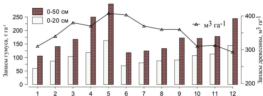
Рис. 3. Запасы гумуса в почвах в слое 0–20 и 0–50 см и запасы древесины кедра.
