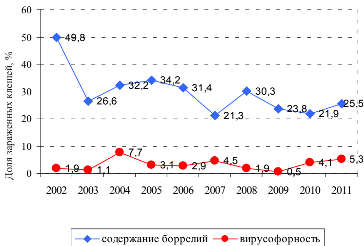
Рис. 2. Заражённость собранных с растительности иксодовых клещей вирусом КЭ и боррелиями в Томском районе
