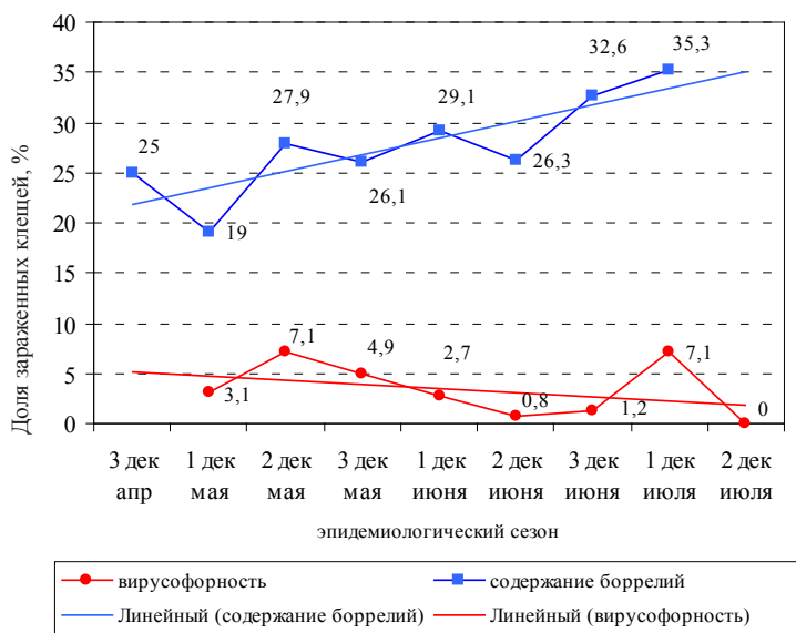
Рис. 3. Изменение заражённости иксодовых клещей вирусом КЭ и боррелиями в течение эпидемиологического сезона
