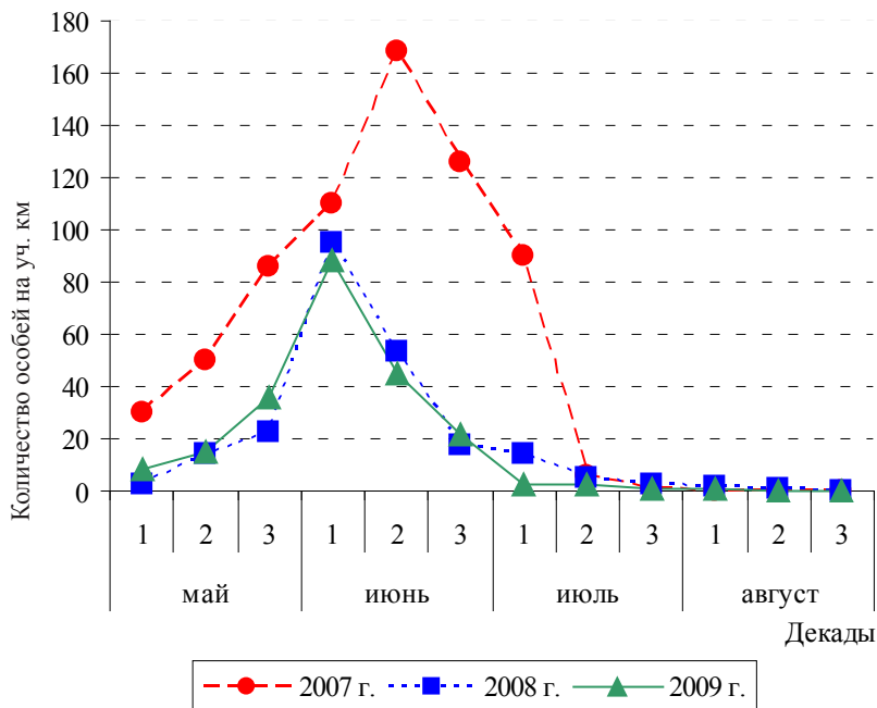
Рис. 1. Динамика активности иксодовых клещей в окрестностях с. Коларово в 2007–2009 гг.
