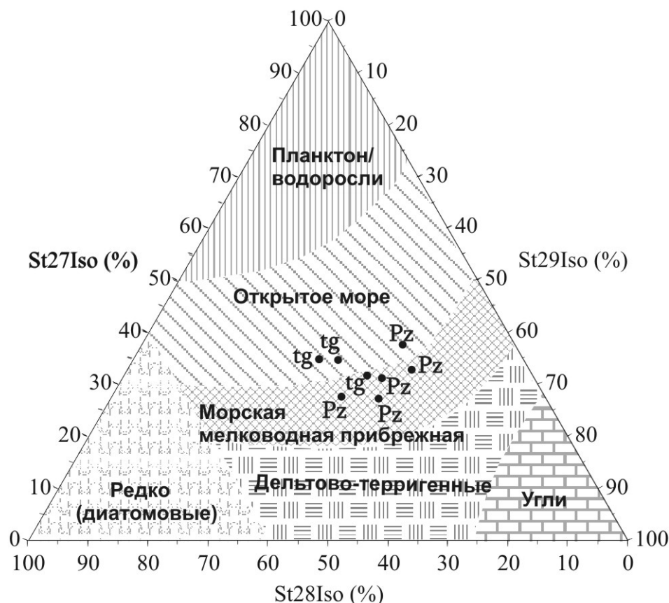
Рис. 4. Распределение изостеранов в исследованных ПОВ (интерпретация в соответствии с Huang & Meinshein [26])
