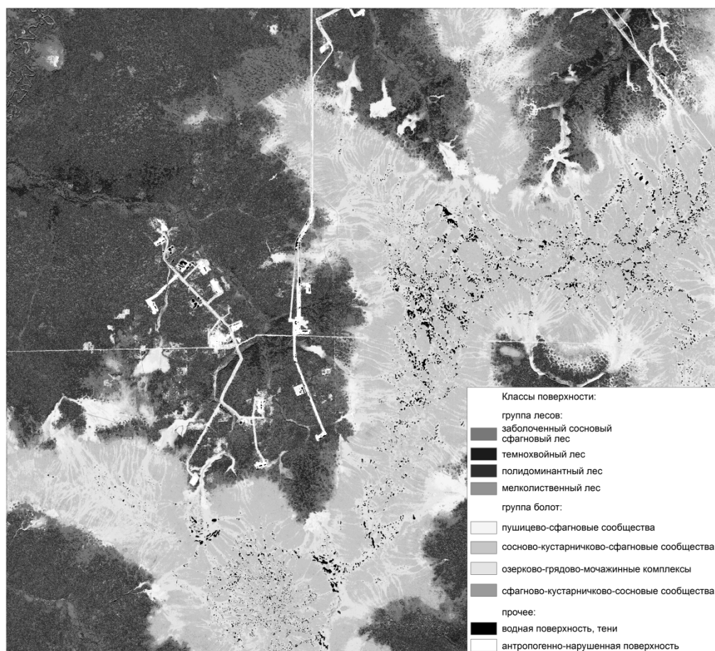
Рис. 1. Классифицированный КС RapidEye, территория ключевого участка
