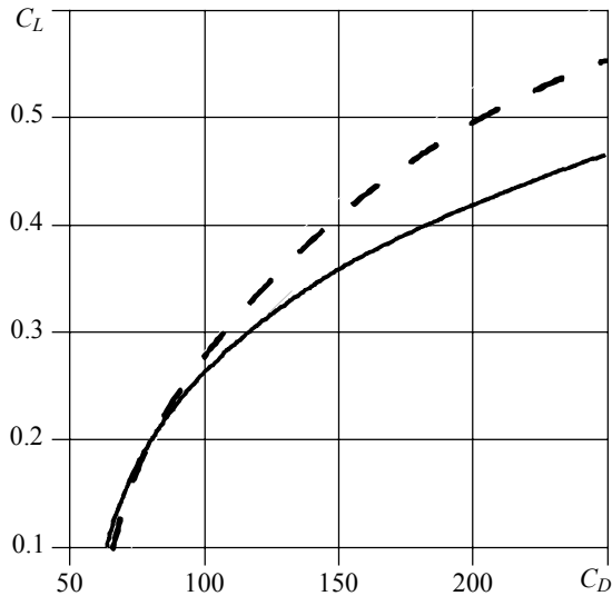
Рис. 1. Поляры (Подъемная сила / Сила сопротивления) при M = 0,75 Fig. 1. Drag polar (ratio of the lift force to the drag force) at M = 0.75
