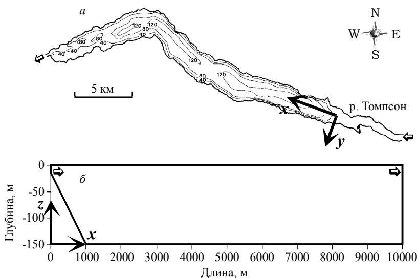
Рис. 2. Озеро Камлупс: a – батиметрия, б – вычислительная область Fig. 2. Kamloops Lake: ( a ) bathymetry and ( б ) computational domain
