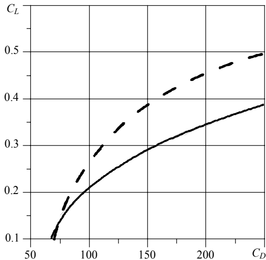
Рис. 2. Поляры (Подъемная сила / Сила сопротивления) при M = 0,8 Fig. 2. Drag polar (ratio of the lift force to the drag force) at M = 0.8
