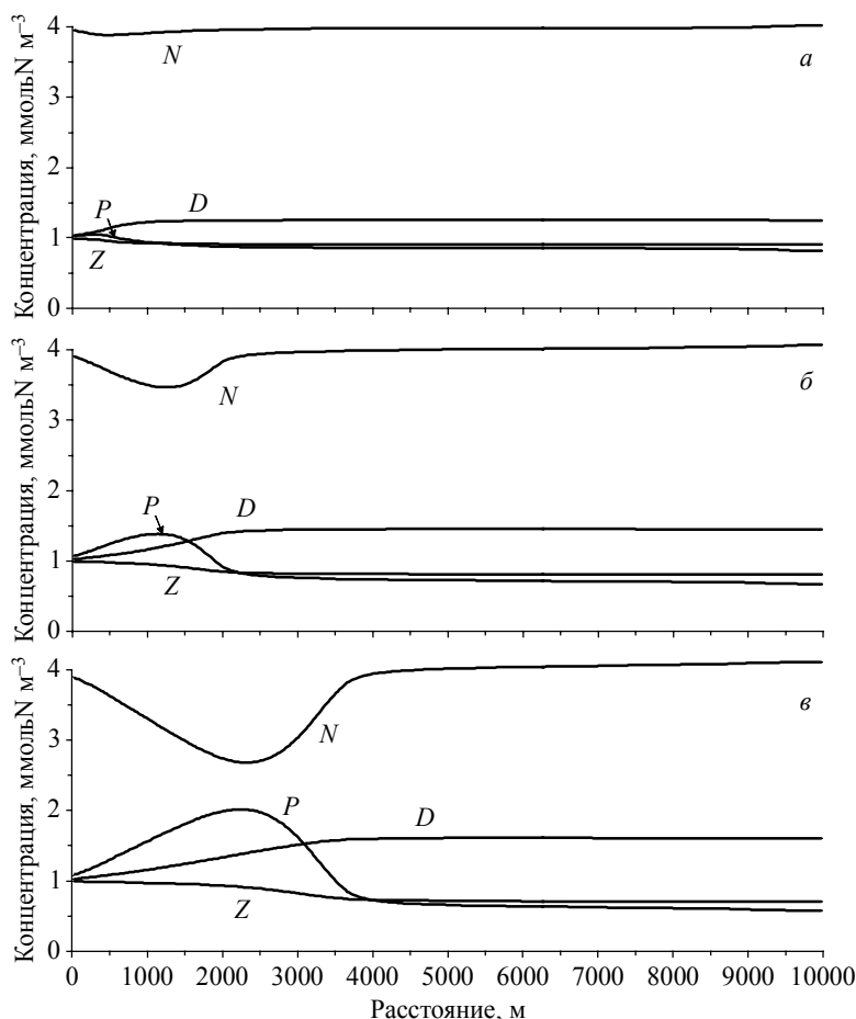
Рис. 3. Профили фито-, зоопланктона, нутриента и детрита на 8 (а), 16 (б) и 24 (в) сутки на глубине 4.5 м Fig. 3. Profiles of phytoplankton, zooplankton, nutrient, and detritus after (а) 8, (б) 16, and (в) 24 days at 4.5 m depth
