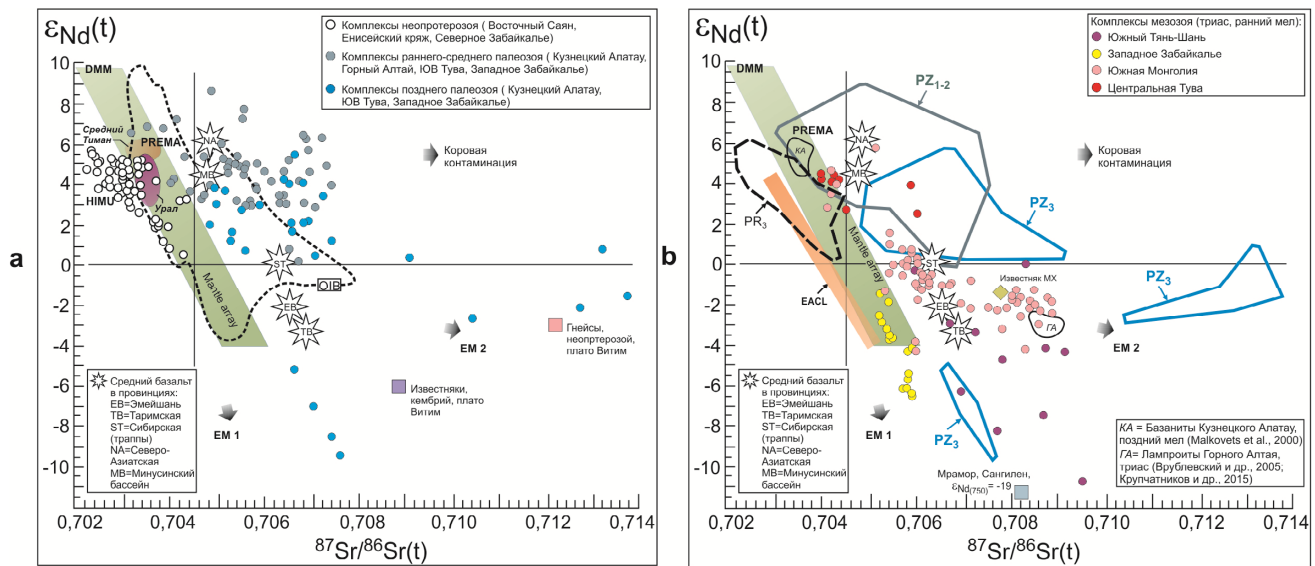
Рис. 3. Изотопный состав неодиума и стронция изверженных щелочных пород и карбонатитов докембрия и палеозоя (а), мезозоя (б) в складчатых областях Северной и Западной Азии
