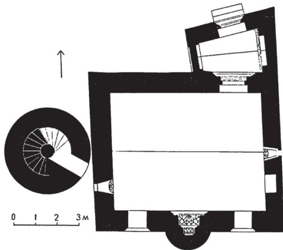
Рис. 3. Мечеть Мухаммеда в Баку (Сыныг-гала, XI в.). План (по Л. Бретаницкому [22. С. 379, рис. 7])
