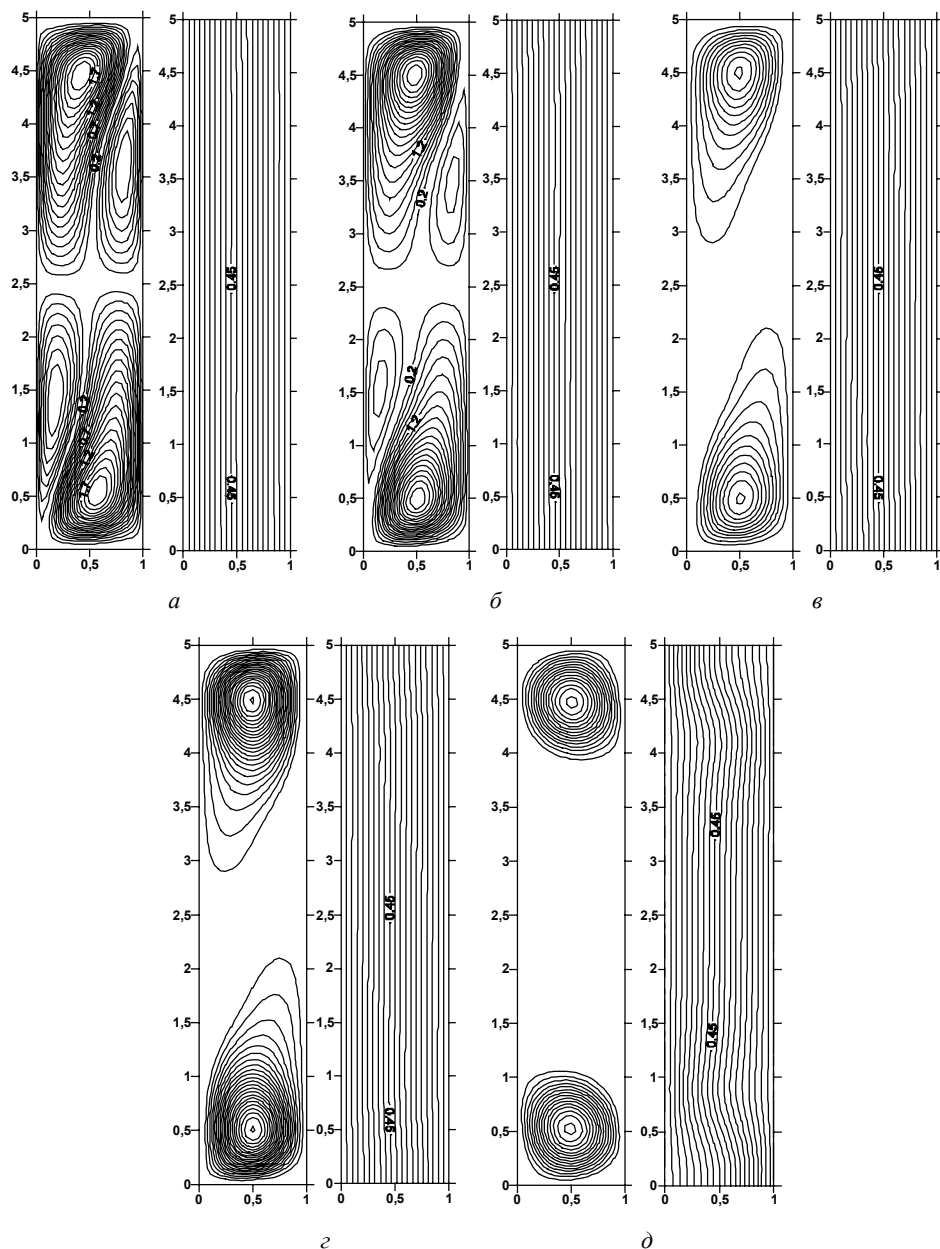
Рис. 1. Изолинии функции тока и температуры при Pr = 0,01 , \alpha = 45^\circ , Gv_a = 2 , Re_{pa} = 10 ; Gv_f : a – 20000; б – 40000; в – 56000; г – 115000; д – 1000000
