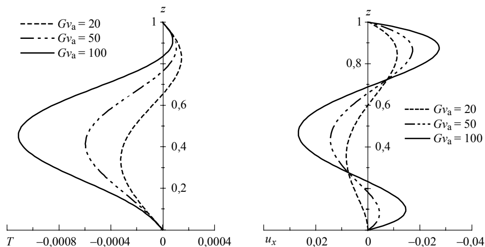
Рис. 6. Профили температуры и скорости аналитического решения при Gr = 1
