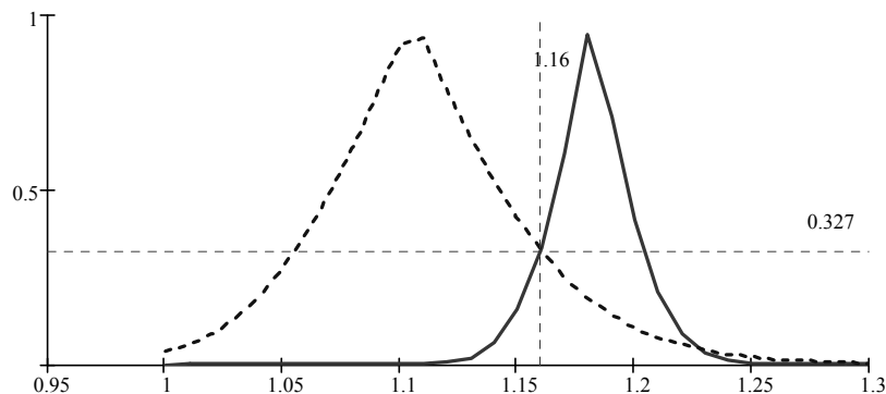
Рис. 3. Точка пересечения критериев Стьюдента и Фишера на примере сравнения изменчивости охвоенности побегов прошлого и текущего годов сосны сибирской
