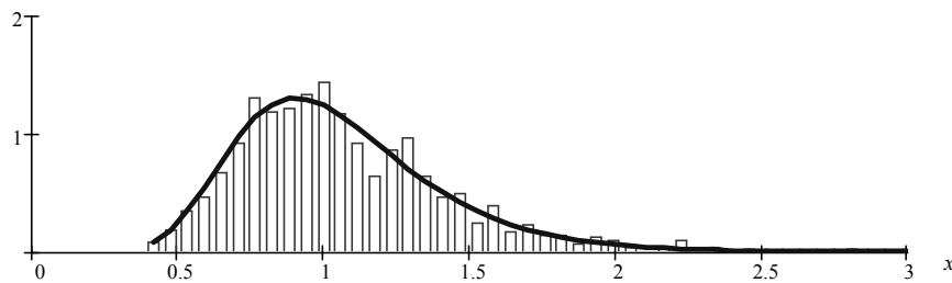
Рис. 1. Гистограмма отношения (1.4) и его теоретическая функция плотности
