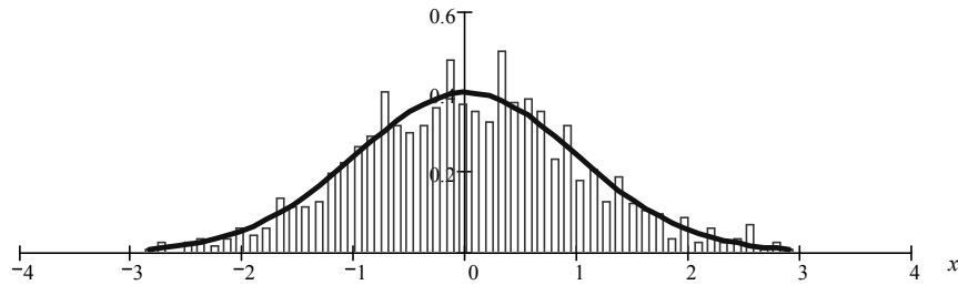
Рис. 2. Гистограмма отношения (1.5) и его теоретическая функция плотности
